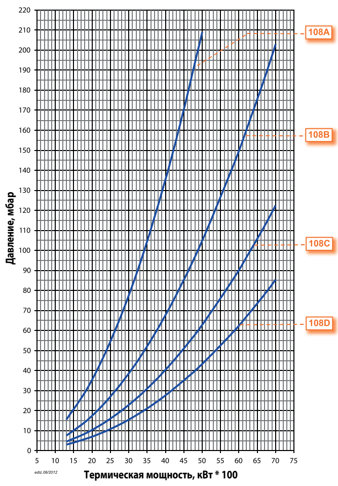
Потери напора (сопловая сборка + газовая рампа) GI 700 DSPGN ME ПРИРОДНЫЙ ГАЗ
