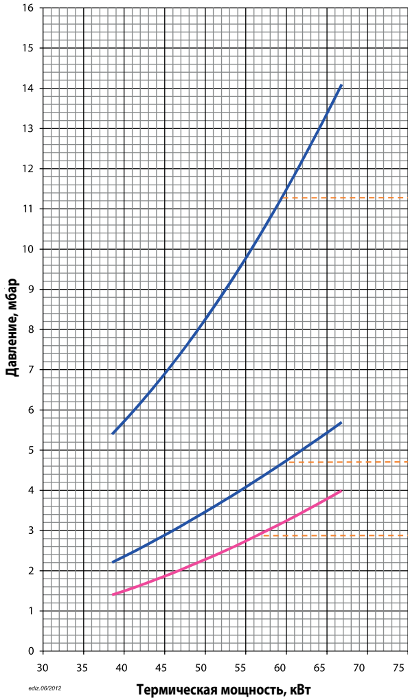
Потери напора (сопловая сборка + газовая рампа)
