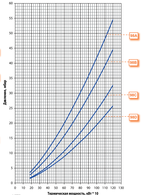
Потери напора (сопловая сборка + газовая рампа) TBG 110 LX ME ПРИРОДНЫЙ ГАЗ
