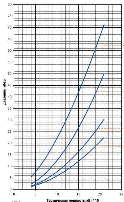
Потери напора (сopловая сборка + газовая рампа)
