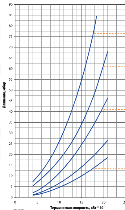
Потери напора (сopловая сборка + газовая рампа)
