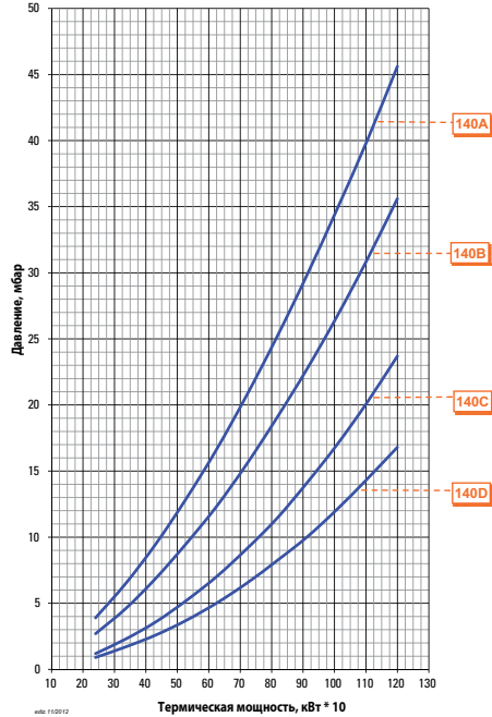
Потери напора (сопловая сборка + газовая рампа) TBG 120 MC ПРИРОДНЫЙ ГАЗ
