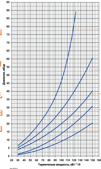
Потери напора (сопловая сборка + газовая рампа) TBG 150PN ПРИРОДНЫЙ ГАЗ
