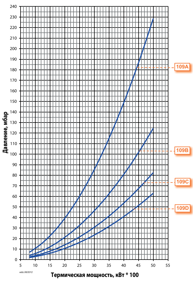
Потери напора (сопловая сборка + газовая рампа) GI 500 DSPGN ME ПРИРОДНЫЙ ГАЗ
