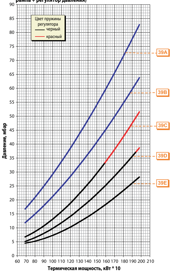
Потери напора (сопловая сборка + газовая рампа)
