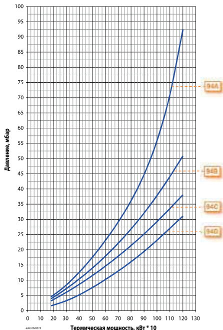
Потери напора (сопловая сборка + газовая рампа) TBG 110 LX PN ПРИРОДНЫЙ ГАЗ
