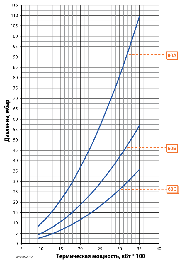
Потери напора (сопловая сборка + газовая рампа) BGN 350 DSPGN ME ПРИРОДНЫЙ ГАЗ
