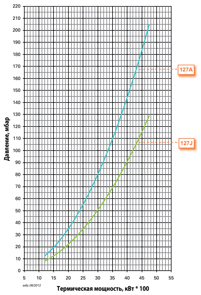
Потери напора (сопловая сборка + газовая рампа) GI 350 DSPGN ПРИРОДНЫЙ ГАЗ
