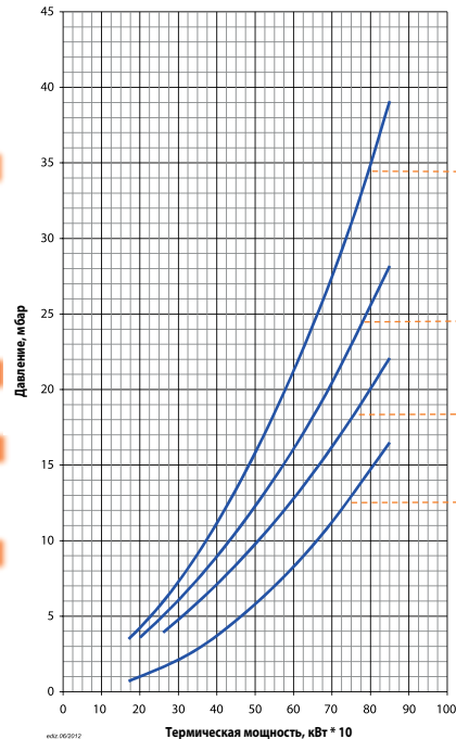
Потери напора (сопловая сборка + газовая рампа)
