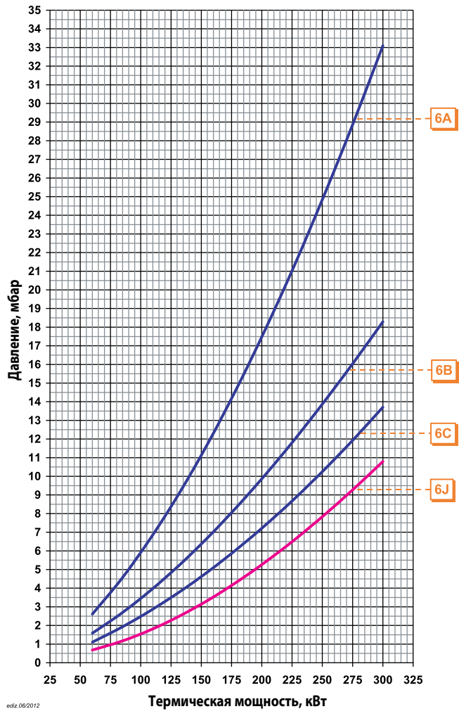
Потери напора (сопловая сборка + газовая рампа) SP ARKGAS 30/30W ПРИРОДНЫЙ ГАЗ
