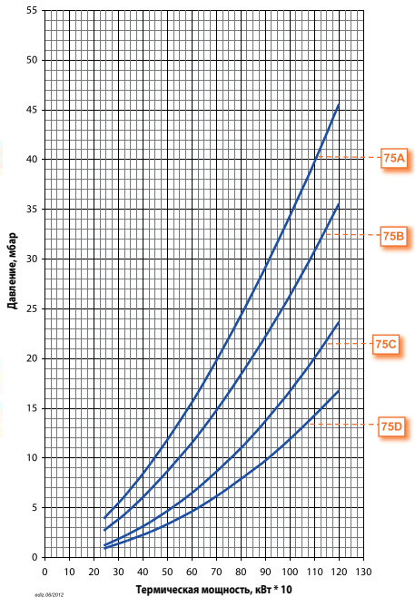
Потери напора (сопловая сборка + газовая рампа) TBG 120 ME ПРИРОДНЫЙ ГАЗ
