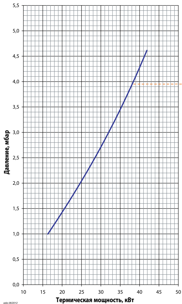
Потери напора (сопловая сборка + газовая рампа)
