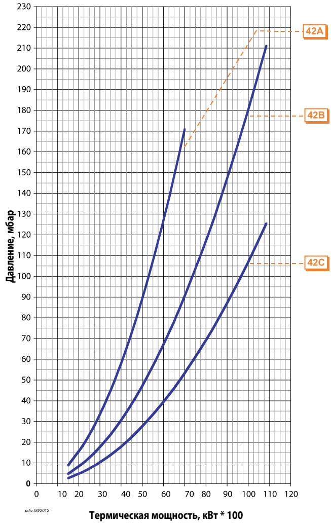
Потери напора (сопловая сборка + газовая рампа) GI 1000LX ПРИРОДНЫЙ ГАЗ
