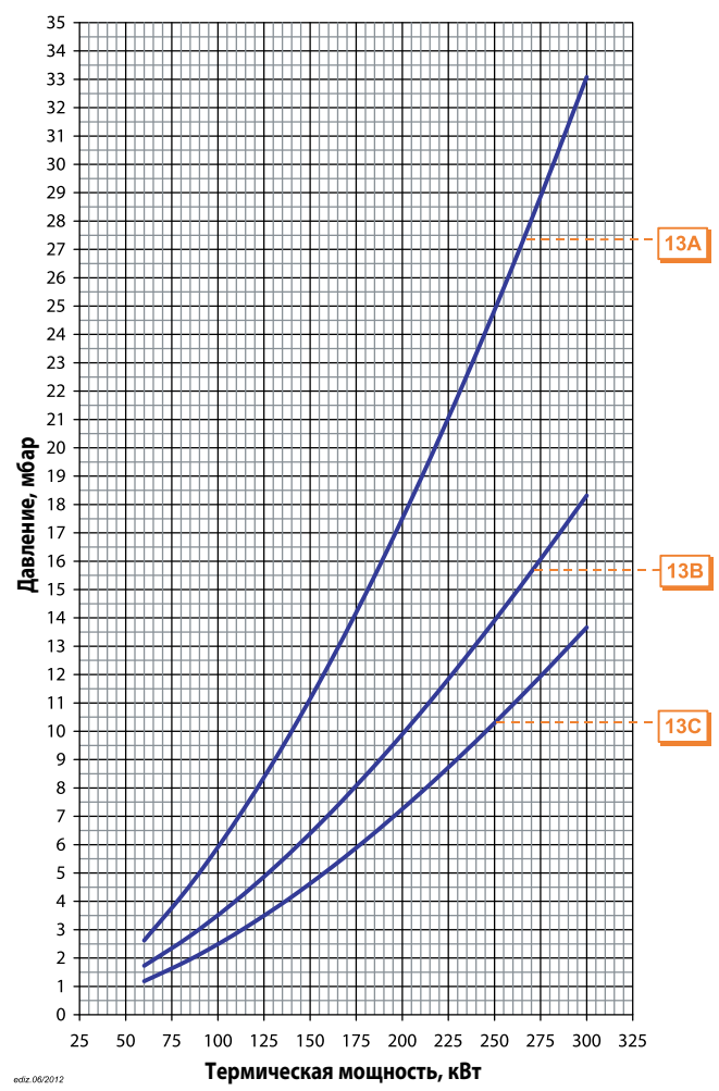
Потери напора (сопловая сборка + газовая рампа) SP ARKGAS 30P/30PW ПРИРОДНЫЙ ГАЗ
