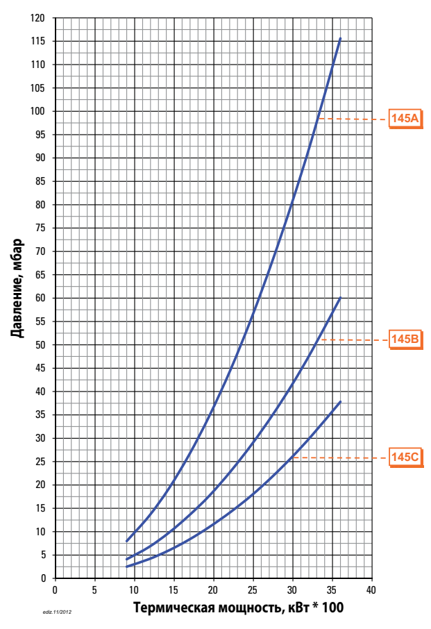
Потери напора (сопловая сборка + газовая рампа) BGN 350 MC ПРИРОДНЫЙ ГАЗ
