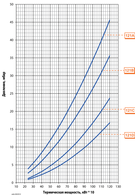
Потери напора (сопловая сборка + газовая рампа) TBG 120 P ПРИРОДНЫЙ ГАЗ
