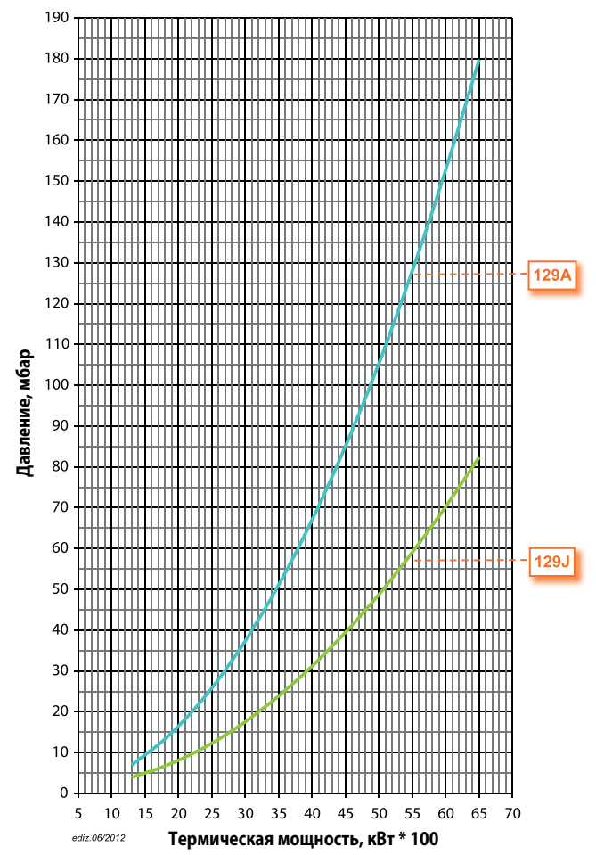
Потери напора (сопловая сборка + газовая рампа) GI 510 DSPGN ПРИРОДНЫЙ ГАЗ
