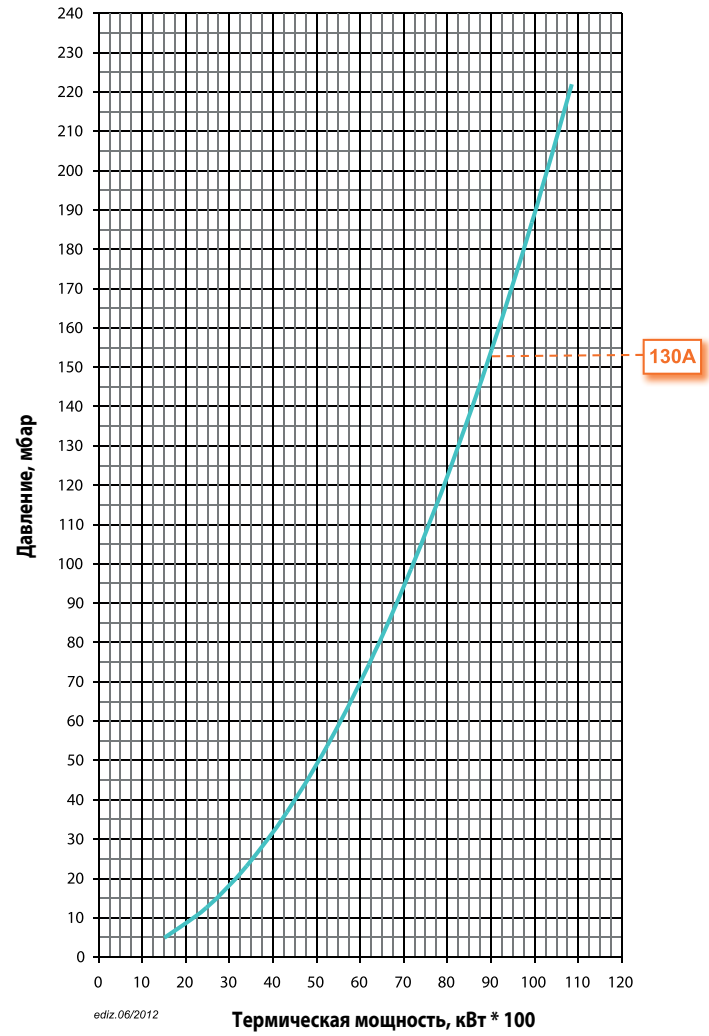
Потери напора (сопловая сборка + газовая рампа) GI 1000 LX ME ПРИРОДНЫЙ ГАЗ
