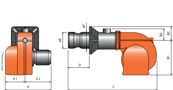
GI 700 DSPGN ME
