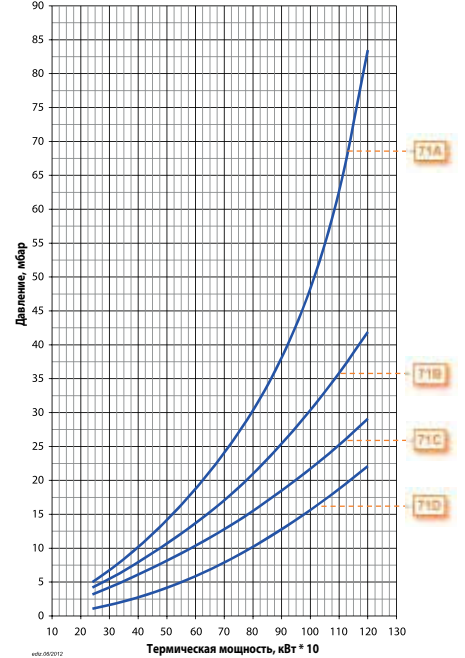
Потери напора (сопловая сборка + газовая рампа) TBG 120PN ПРИРОДНЫЙ ГАЗ
