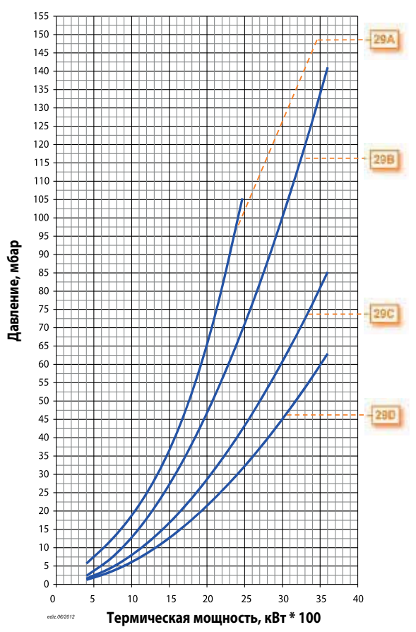
Потери напора (сопловая сборка + газовая рампа) BGN 300 LX ПРИРОДНЫЙ ГАЗ
