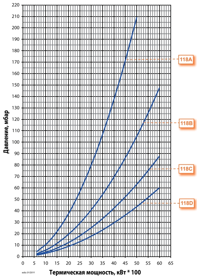
Потери напора (сопловая сборка + газовая рампа)
