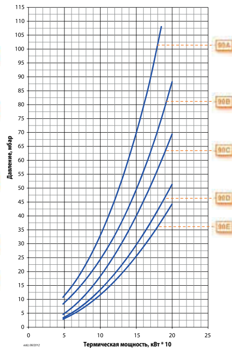
Потери напора (сopловая сборка + газовая рампа)
