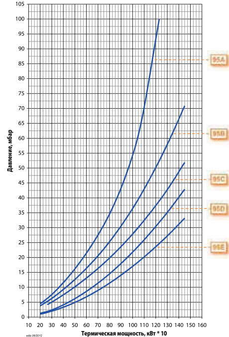
Потери напора (сопловая сборка + газовая рампа) TBG 140 LX PN ПРИРОДНЫЙ ГАЗ
