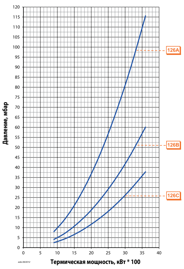
Потери напора (сопловая сборка + газовая рампа) BGN 350 P ПРИРОДНЫЙ ГАЗ
