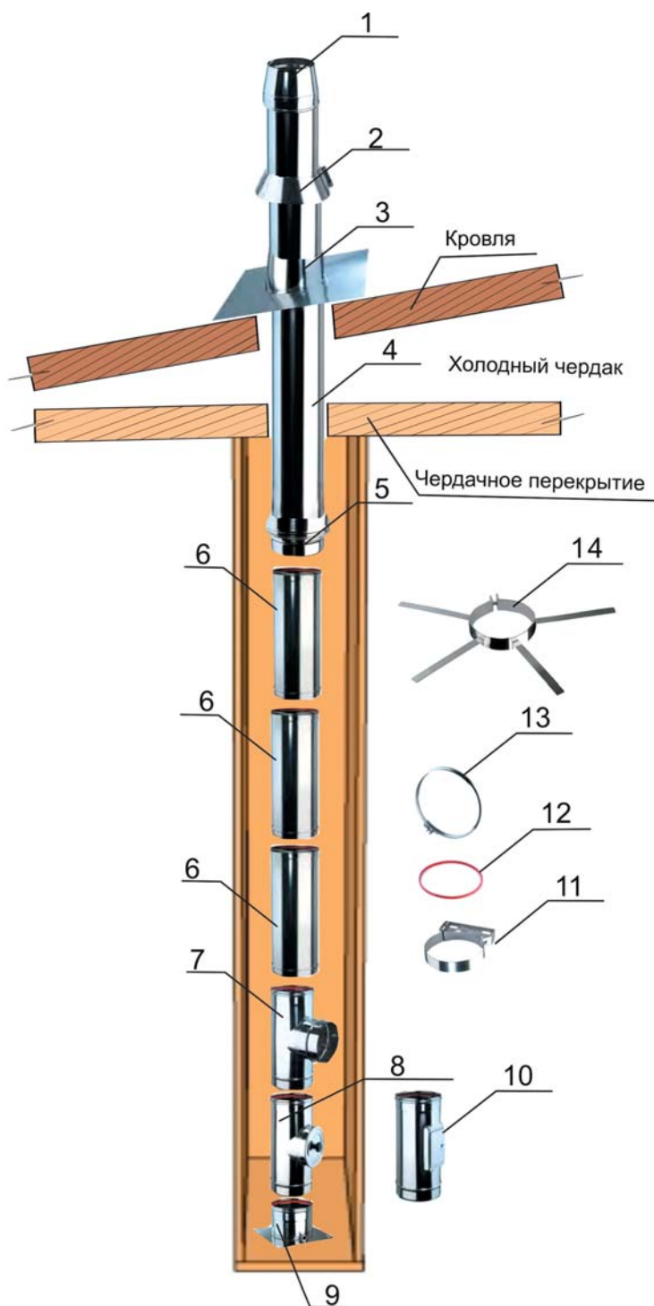
Рисунок 1. Схема поэтапного устройства дымохода, прокладываемого в канале
