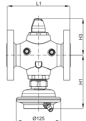
AVPB-F (PN25) DN 32 - 50
