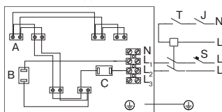
Схема подключения № 2
