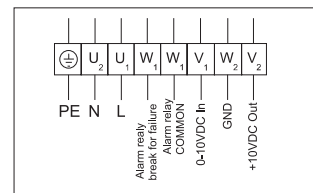
Схема подключения № 2
