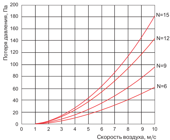
Рис. 2. График падения давления в нагревателе
