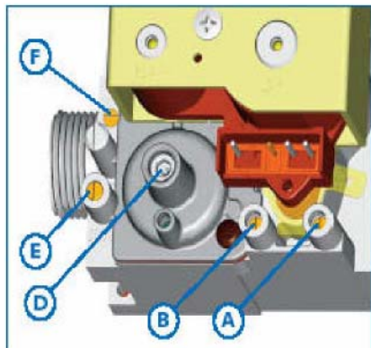
Рис. 5.4 Газовый мультиблок Sigma 848
