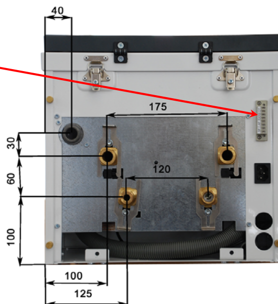
Вид снизу: Размеры для подключения
