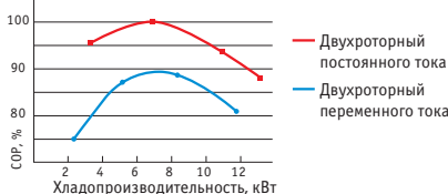
Энергоэффективность компрессора
