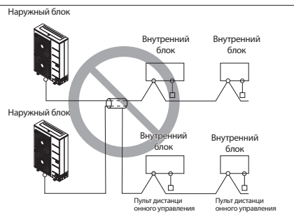
Многожильный кабель
