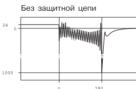
Осциллограммы напряжения на катушке при отключении
