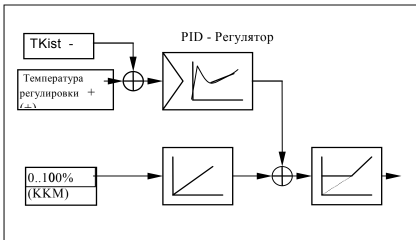
Рис.: Принципиальная схема управления мощности с помощью котлового модуля горелки в каскаде.
