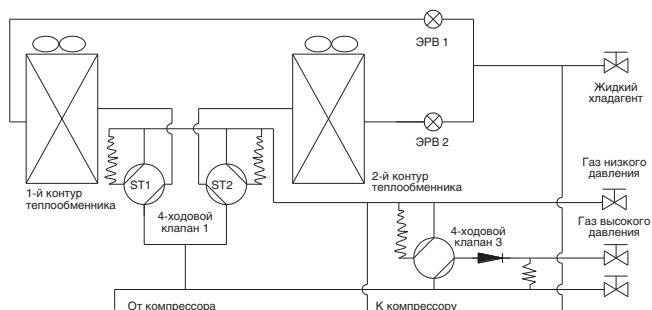
Гидравлическая схема. Два независимых контура теплообменника.
