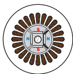
Централизованная обмотка
