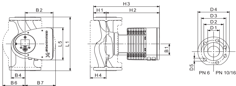
Рис. 51 Габаритные размеры, одинарные насосы, фланцевая версия
