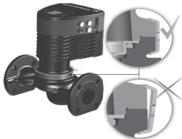
Рис. 17 Закрепление головной части насоса на корпусе
