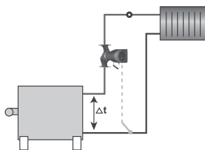
Рис. 38 Перепад температур
