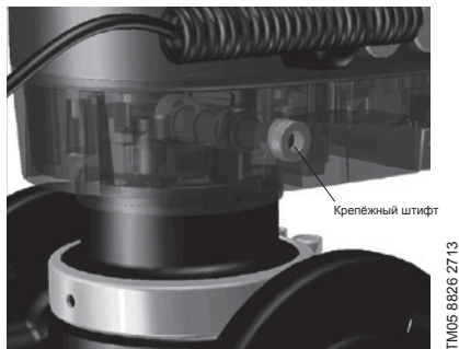
Рис. 12 Крепёжный штифт для модификаций с подключением через штекер
