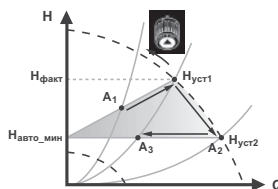
Рис. 31 AUTO_{ADAPT}
