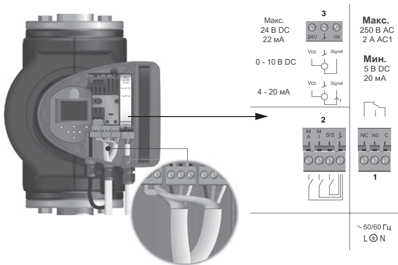
21-сур. Қосылым сызбасы, клемма арқылы түрленім
