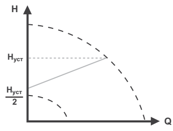
33-сур. Пропорционалды қысым
