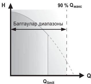
Рис. 41 FLOW LIMIT
