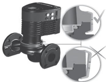
17-сур. Корпуста сорғының басқы бөлігін бекіту
