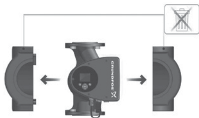
Рис. 4 Теплоизоляционные кожухи
