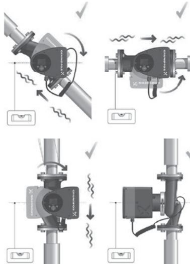
14-сур. Көлденең күйіндегі басқару блогты сорғы
