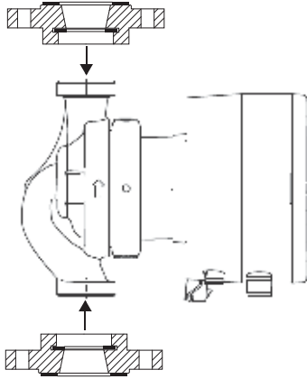
Սկար 39 Կցաշտրթային պարտրակավոր հարմարակցիչների օրինակ
