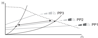
25-сур. Қысымды тепе-тең өлшеудің үш қысық басқару режимдері
