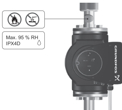
Рис. 11 Перекачиваемые жидкости
