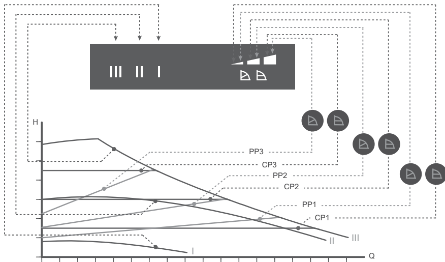
24-сур. Соркысманын жумушчу мүнөздөмөлөрүнө жараша башкаруу шарттамдары
