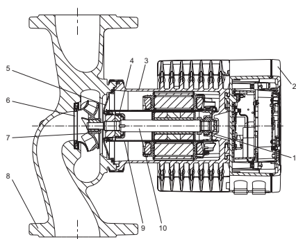
Рис. 1 Исполнение с подключением питания к клеммам внутри электронного блока, гильзой ротора из PPS и фланцевым соединением
