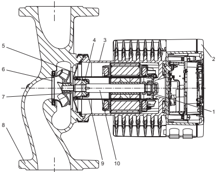
Նկար 1 Կատարում, որտեղ սնուցումն էլեկտրոնային բլոկի ներսում միացված է սեղմակների, PPS-ից պատրաստված ռոտորի պարկույծով և կցաշրջային միացմամբ
