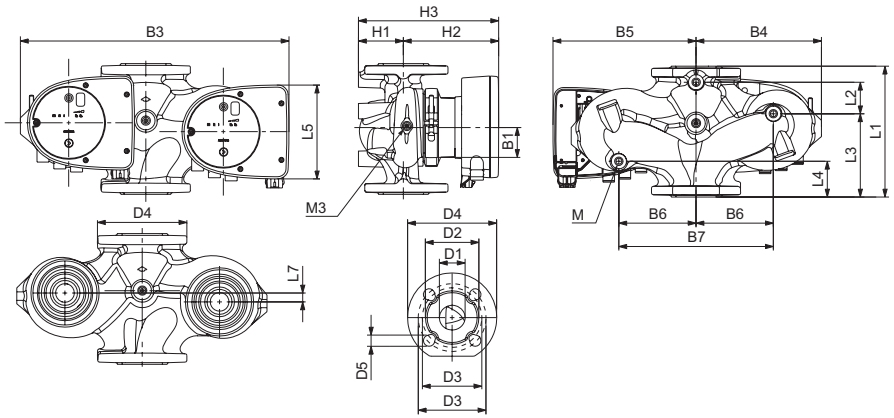
Նկար 48 Ջույգ պոմպերի գաբարիտային չափսերը, կատարում կցաշտրթային միացքով և սնուցման շտեկերային միացումով
