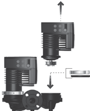
Նկար 36 Փակ կցաշուրթի տեղադրում
