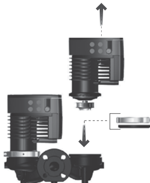
36-сүр. Туяк фланецти онотуу
