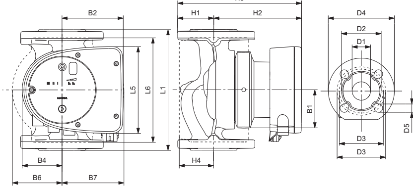
Նկար 46 Միայնակ պոմպերի գաբարիտային չափերը, կատարում կցաշրջության միացքով և սնուցման շտեկերային միացումով
