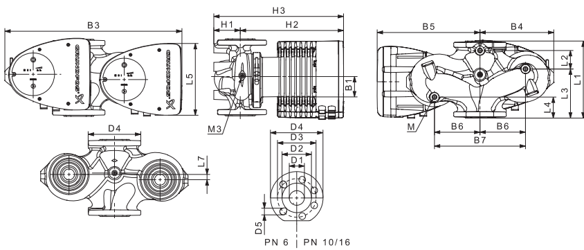
Նկար 49 Չույգ պոմպերի գաբարիտային չափերը, կատարում կցաշորթային միացրով և ստուցման սեղմակային միացումով
