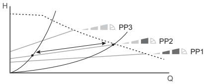
Նկար 25 Ճնշման համեմատական փոփոխության ռեժիմի երեք կորերը
