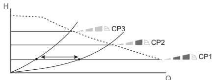
26-сур. Қысымның тұрақты мәнiмен үш қысық басқару режимдері
