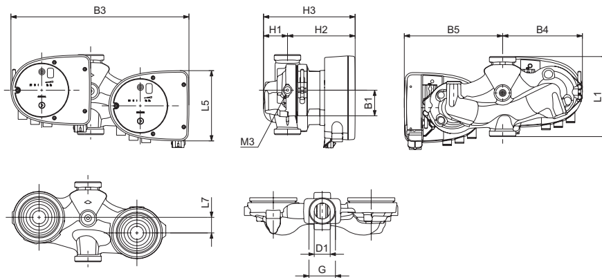
45-сүр. Эки катар соркысмардын тыш өлчөмдөрү, сайлык бириктирүү аткаруусу
