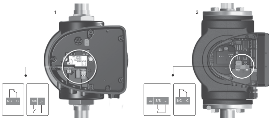
Рис. 22 Подключение к внешнему управлению
