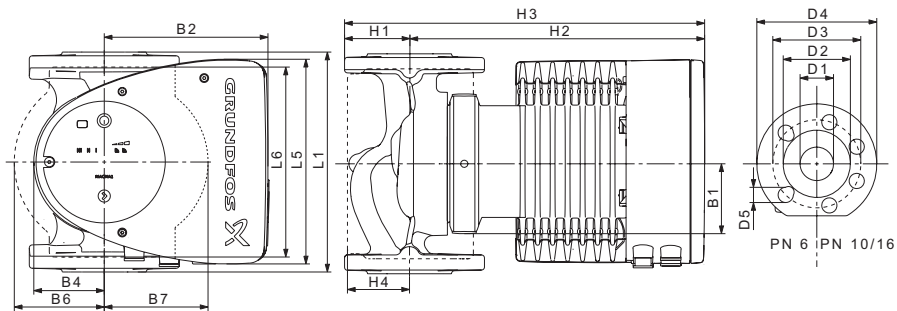
47-сүр. Бир қатар сорқысмалардын тыш өлчөмдөрү, фланецтик бириктирүү жана клеммалар аркылуу азыкты туташтыруу менен аткаруу
