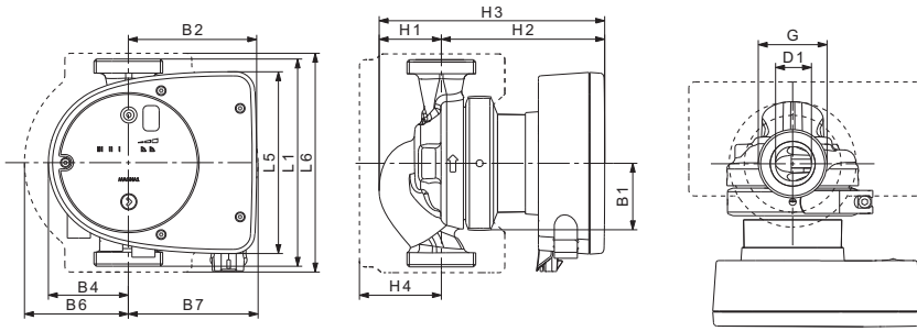
Նկար 44 Միանակ պոմպերի գաբարիտային չափերը, կատարում պարուրակավոր միացումով
