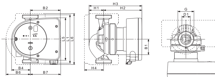
44-сүр. Бир катар соркысмардын жалпы көлөмү, оймо туташтыруу менен аткаруу
