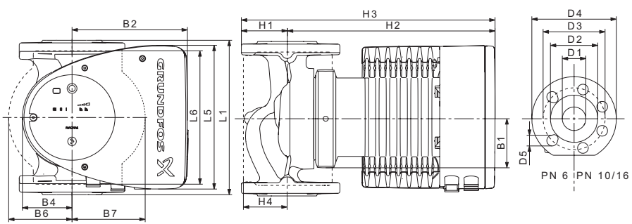
Նկար 47 Միայնակ պոմպերի գաբարիտային չափսերը, կատարում կցաշուրթային միացրով և սնուցման սեղմակային միացումով
