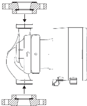
39-сур. Фланецтік-резьбалық жалғастырғыш тетіктер мысалы
