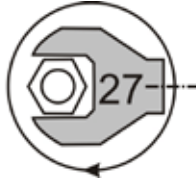
1 (360°) Тип резьбы G 3/4 *1 6098 xx
