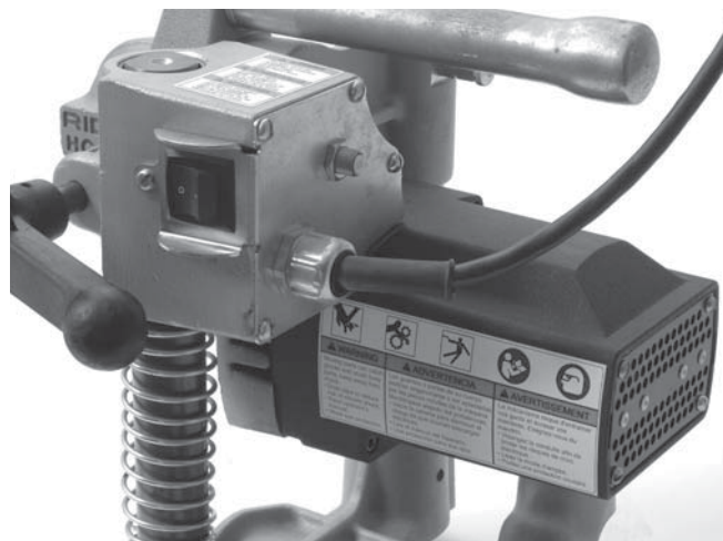
Figur 4B – HC-300-advarselmærkater
