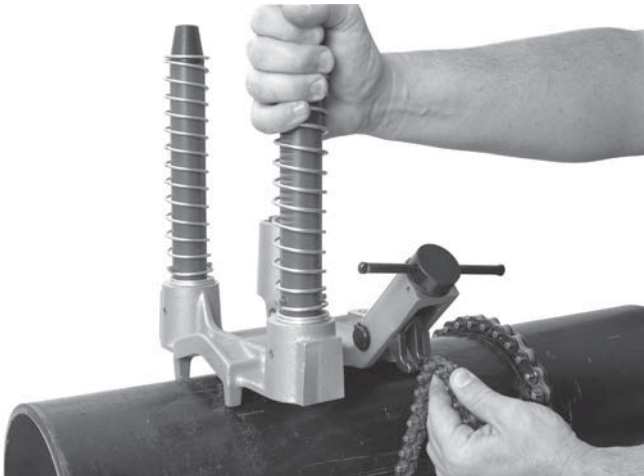
Kuva 8 – Ketjun kiinnitys
