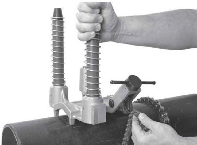
Rysunek 8 – Zahaczanie łańcucha
