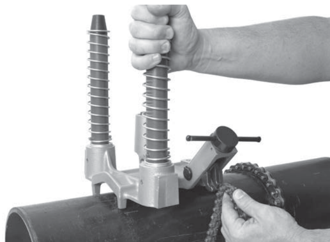
Рис. 8 - Крепление цепи
