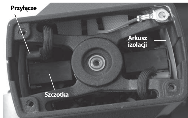
Rysunek 12 – Umieszczenie szczotek - zdjęta pokrywa silnika
