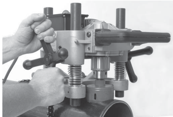
Figure 11 – Utilisation de la scie à cloche
