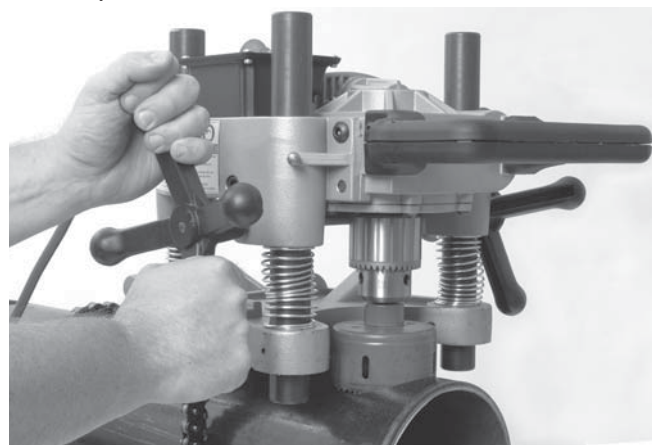
Slika 11 – Rad alata za izrezivanje rupa
