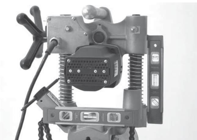
Рис. 10 – Выравнивание станка HC-300
