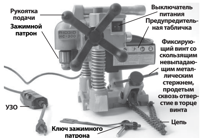
Рис. 2 – Модель HC-300 со стандартными принадлежностями
