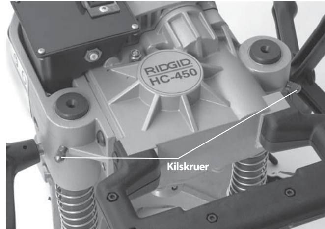
Figur 13 – Justere kilskruer
