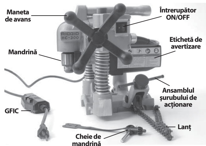
Figura 2 – Model HC-300 cu echipamentul standard
