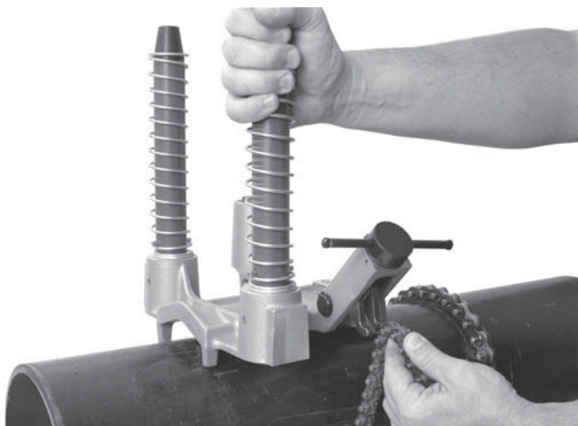
Slika 8 – Zakvačivanje lanca
