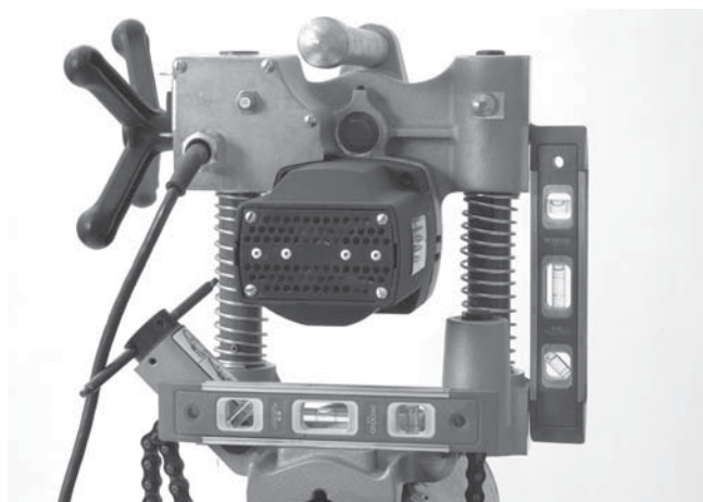
Obrázek 10 – vyrovnání modelu HC-300
