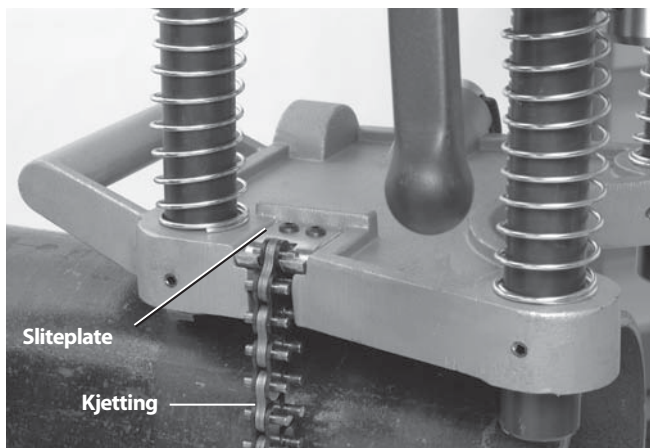
Figur 5 – Feste HC-450-kjettingen
