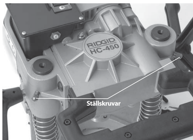
Figur 13 – Justera ställskruvarna
