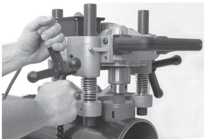
Figuur 11 – Bedienen van de gatzaagmachine
