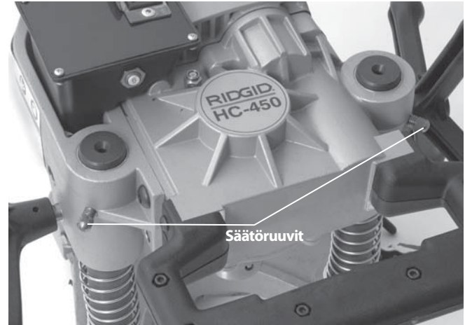
Kuva 13 – Säätöruuvien säätö
