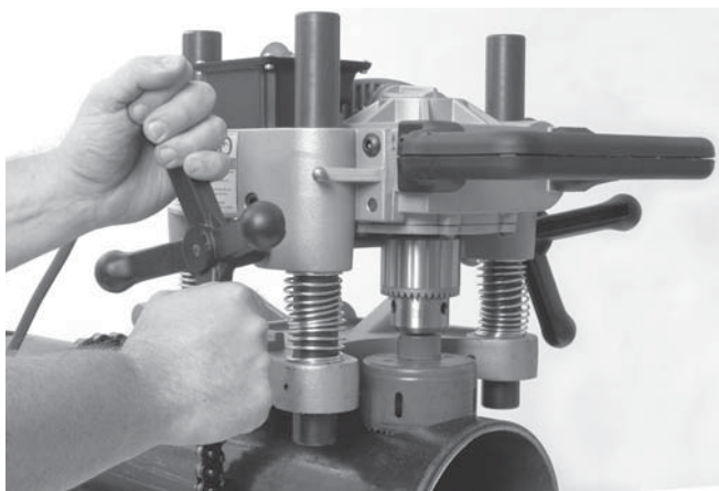
Figura 11 – Acționarea dispozitivului de perforare
