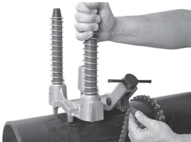
Slika 8 – Kačenje lanca
