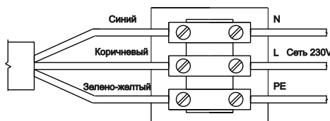
Рис.7 Схема подключения ETT (EI.05E)
