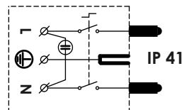
Сн.8 Схема на свързване на VS1 VS1
