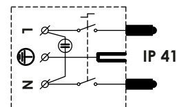
Rys.8 Schemat podłączenia VS 1
