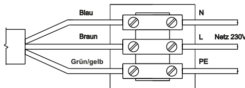
Abb. 7 Schaltplan des EHK (EI.05E)
