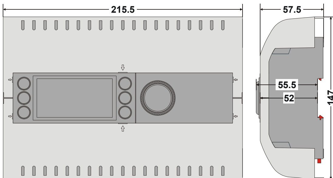
Рис. 6. Размеры контроллера MVC с дополнительными панелями (в мм.)
