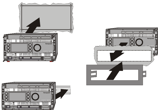
Рис. 3. Варианты монтажа
