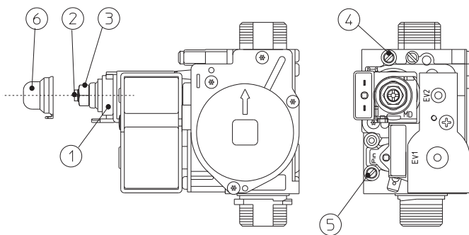
Zawór Gazu SIT 845
