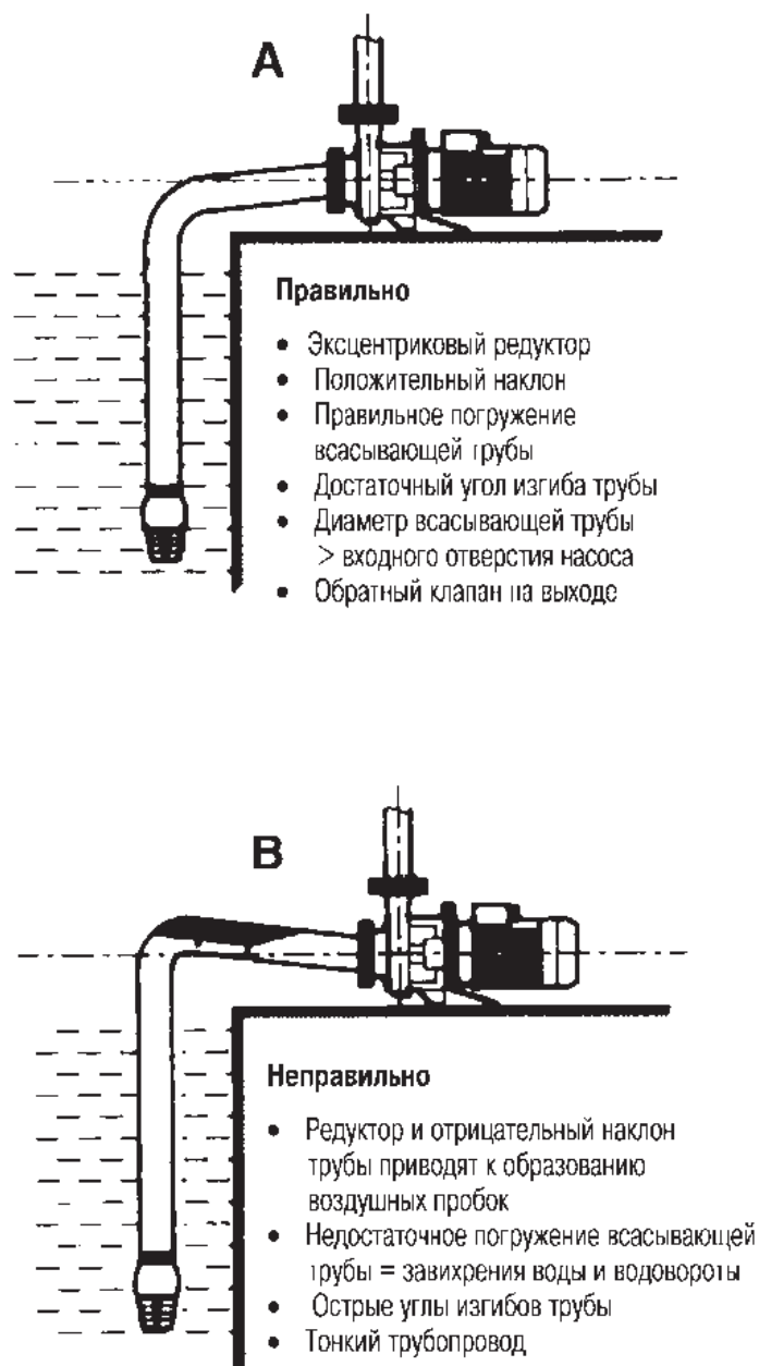
Рис. 1 – Установка насоса
