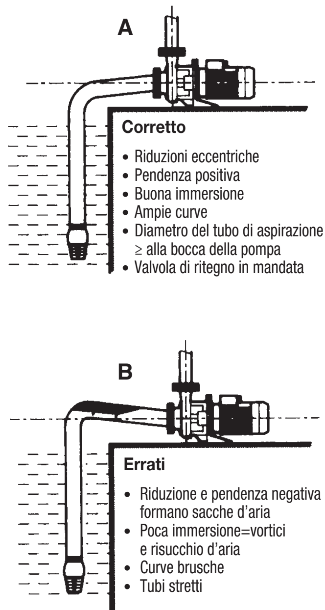
fig. 1 - schema installazione
