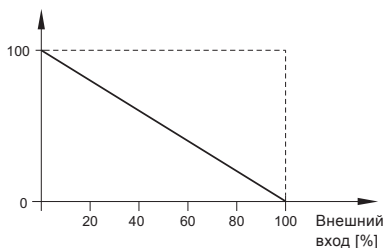
Рис. 59 Обратная функция
