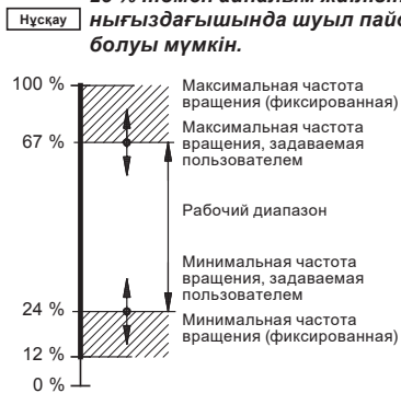
55-сур. Мейлінше жоғары және мейлінше төмен орнатылым мысалы
