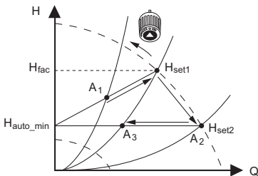
Рис. 36 AUTO ADAPT
