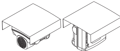
Рис. 11 Примеры защитных кожухов (не поставляются компанией Grundfos)
