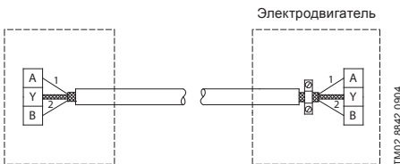
27-сур. Экрандалған екі тармақты кабельді жалғау
