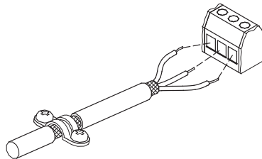
25-сур. Экраны мен сымды жалғаулары бар тазартылған кабель.
