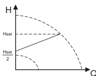
Пропорциональное давление
