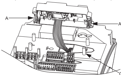
16-сур. Пластмасса қақпақты қайта орнату.
