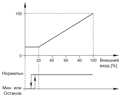
Рис. 58 «Линейно с остановом» или «Линейно с мин.»
