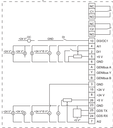
24-сур. Байланыс клеммалары, FM 20
