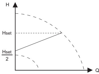
Рис. 38 Пропорциональное давление
