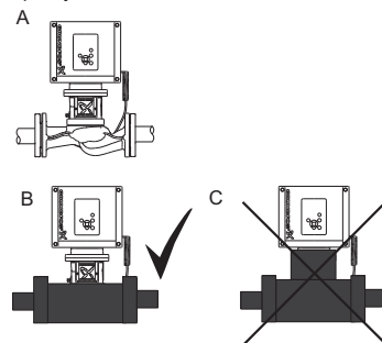
9-сур. TPE2, TPE3 сорғыларын оқшаулау
