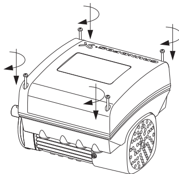
17-сур. Клеммалы қораптың қақпағын орнату
