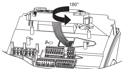
15-сур. Пластмасса қақпақты бұру.
