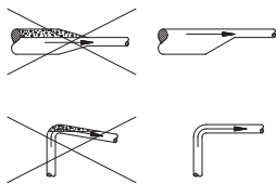
8-сур. Құбыржелісінің сору жағындағы дұрыс конфигурациясы
