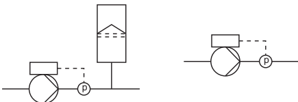
Рис. 41 Постоянное давление
