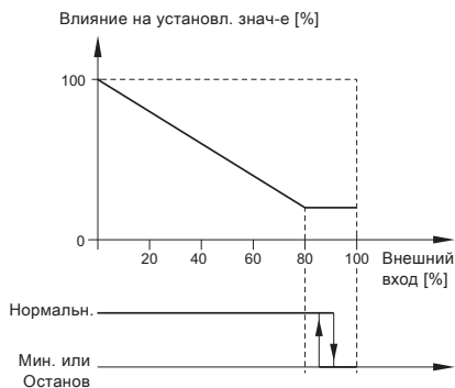
Рис. 60 «Обратно с остановом» (Обратно пропорционально с остановом) и «Обратно с мин.» (Обратно пропорционально с мин.)
