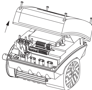
13-сур. Клеммалы қораптың қақпағының шешілуі
