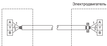
Рис. 26 Подключение 3-жильного экранированного кабеля
