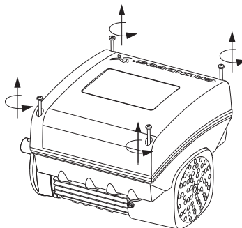
Рис. 12 Отвинчивание винтов
