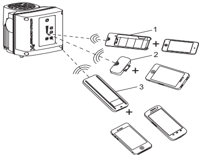
67-сур. Grundfos GO Remote және радио немесе инфрақызыл сигнал арқылы сорғысының арасындағы байланыс
