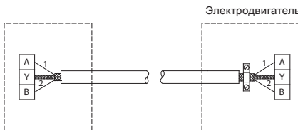
Рис. 27 Подключение 2-жильного экранированного кабеля
