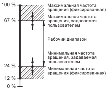
Рис. 55 Пример минимальных и максимальных установок
