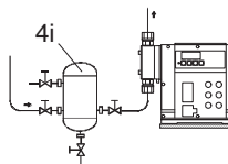
Рис. 10 Установка с демпфером пульсаций давления на всасывающей линии
