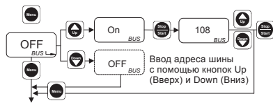
Рис. 56 Активация PROFIBUS для насоса
