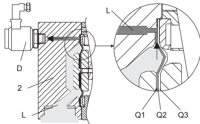
Рис. 2 Дозирующая головка с комплектом мембран и датчиком давления для обнаружения разрыва мембраны
