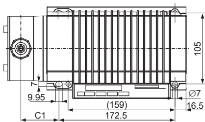
Рис. 4 Схема сверления
