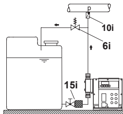
9-сур. Сақтандырғыш клапанымен және сүзгісімен орнату
