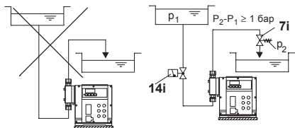
8-сур. Сифонды эффектін болдырмауға арналған қондырғы
