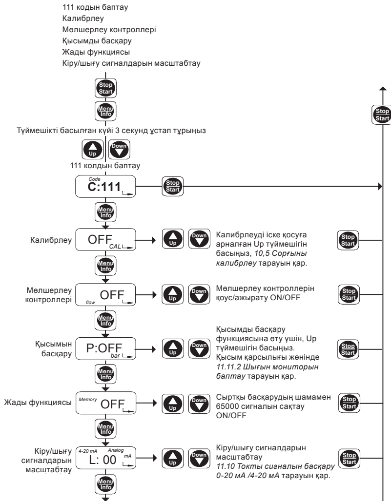
31-сур. Екінші функционалды деңгей, 1-нұсқау бөлімі
