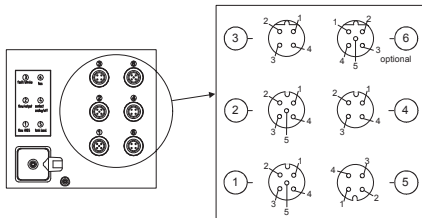
Рис. 16 Подключение к насосу DDI 222
