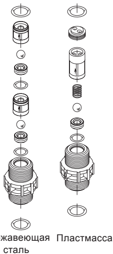
Рис. 57 Клапан из нержавеющей стали или пластмассы в исполнении DN 20, подпружиненный (опция)
