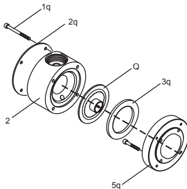
Рис. 60 Замена мембраны для DDI 60-10
