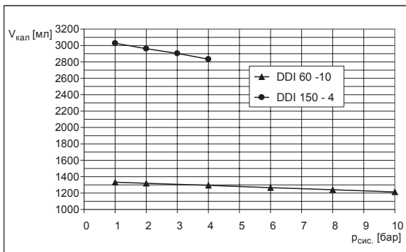
19-сур. Мөлшерлеу өндірімділігінің диаграммасы
