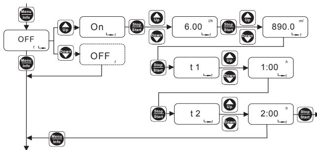
54-сур. Таймер режимін баптау
