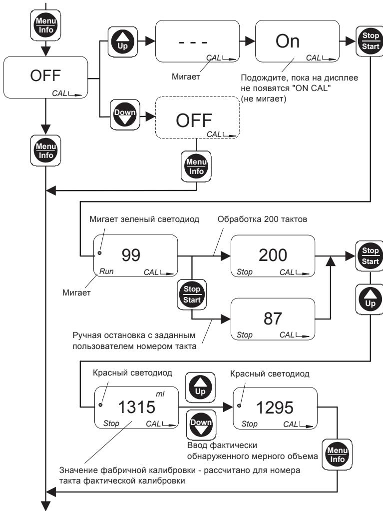
Рис. 18 Калибровка
