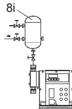
11-сур. Пульстелу қысым бар қондырғы
