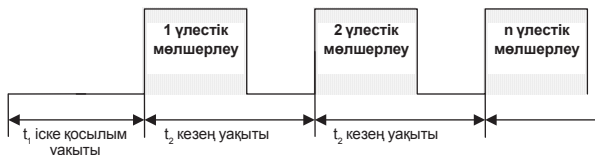
53-сур. Таймер бойынша жұмыс
