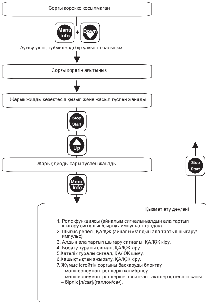
33-сур. Қызмет көрсету деңгейін ашу және одан шығу
