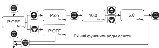
43-сур. Сорғы айырылымын баптау
