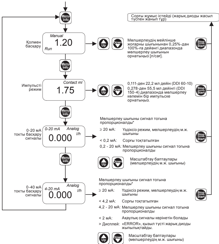
27-сур. Бастапқы функционалды деңгей
