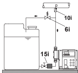
Рис. 9 Установка с предохранительным клапаном и фильтром
