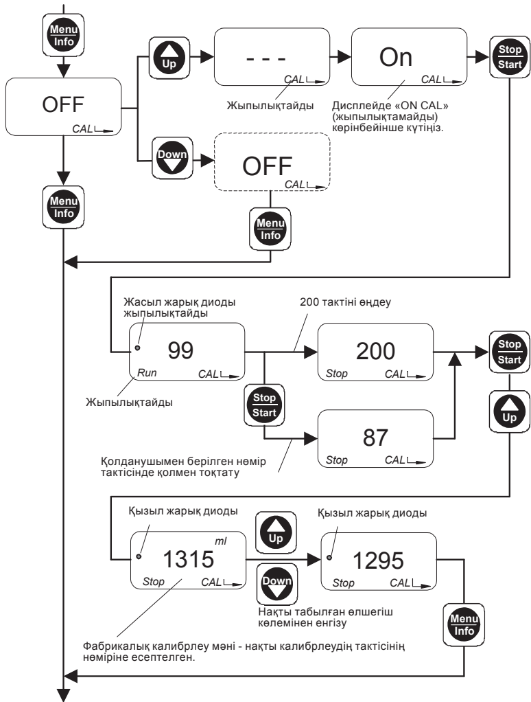
18-сур. Калибрлеу
