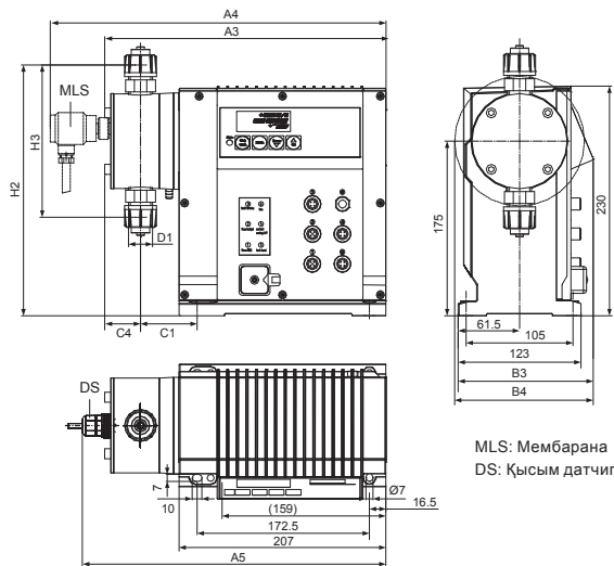
59-сур. Мембрана датчигі бар (алдыңғы көрінісі) және қысым датчигі бар (жоғарғы көрінісі) DDI 222 габаритті өлшемдері
