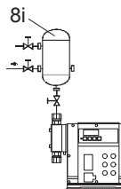
Рис. 11 Установка с демпфером пульсаций давления
