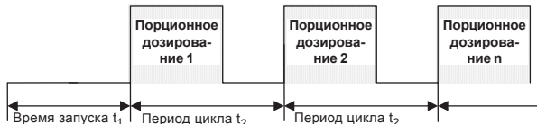
Рис. 53 Работа по таймеру
