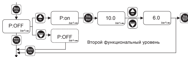
Рис. 43 Настройка отсечки насоса
