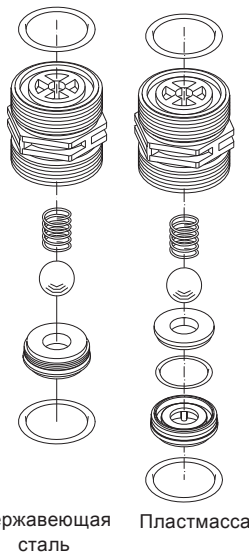
Рис. 58 Клапан из нержавеющей стали или пластмассы в исполнении DN 20, подпружиненный - (опция)
