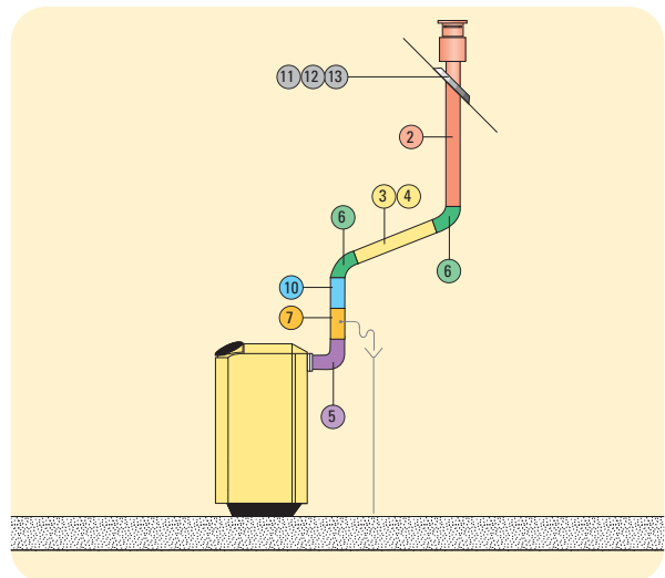
GÉODIS BVi vertical outlet.
