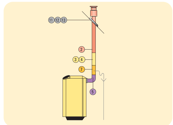
GÉODIS BVi straight roof outlet.
