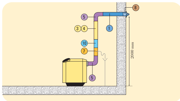
GÉODIS CVi raised horizontal outlet.
