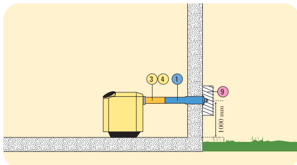
GÉODIS CVi straight wall outlet.
