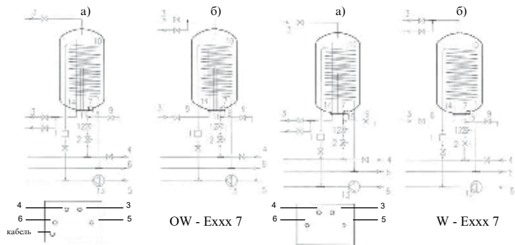
Рис. 5. Схема гидросистемы а) без циркуляции, б) с циркуляцией 1. воздушный клапан, 2. редукционный клапан, 3. теплая вода / вход циркуляции 4. холодная вода, 5. вход теплообменника, 6. выход теплообменника, 7. датчики, 8. циркуляция, 9. воздушный вентиль, 10. змеевик-теплообменник, 11. ТЭН, 12. предохранительный клапан, 13. циркуляционный насос, 14. трубка РЕХ 15. тройник, 16. крышка
