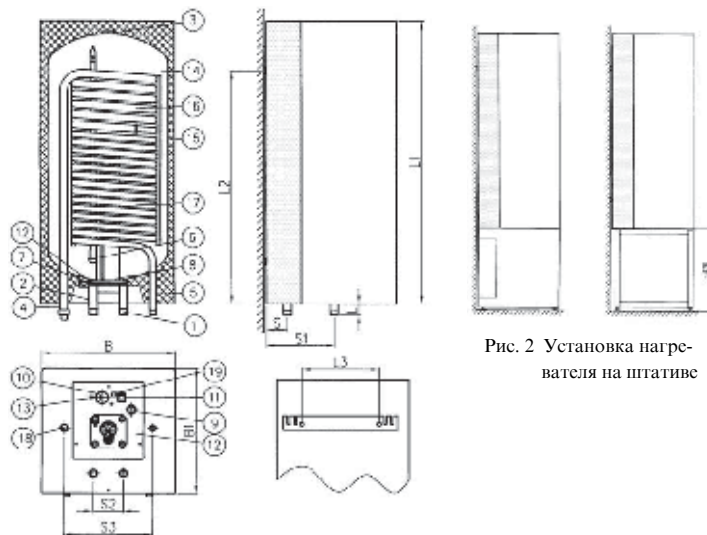
Рис. 1 Конструкция нагревателя
