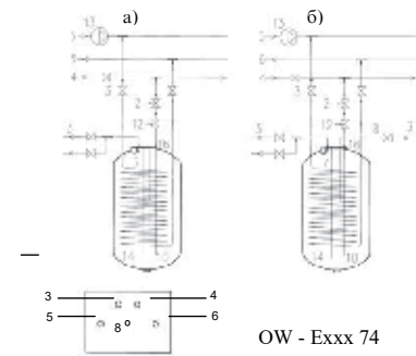
Рис. 5. Схема гидросистемы а) без циркуляции, б) с циркуляцией 1. воздушный клапан, 2. редукционный клапан, 3. теплая вода / вход циркуляции 4. холодная вода, 5. вход теплообменника, 6. выход теплообменника, 7. датчики, 8. циркуляция, 9. воздушный вентиль, 10. змеевик-теплообменник, 11. ТЭН, 12. предохранительный клапан, 13. циркуляционный насос, 14. трубка РЕХ 15. тройник, 16. крышка
