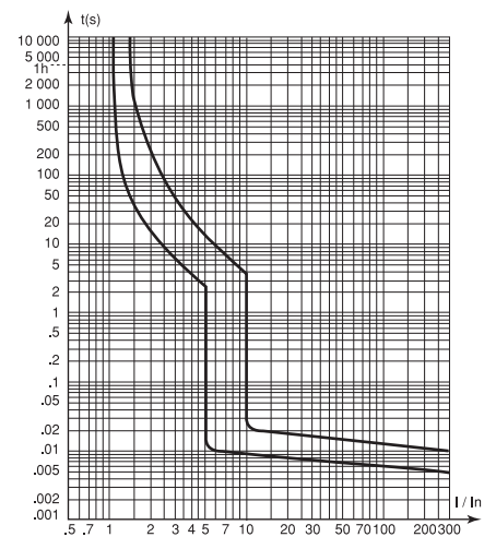
NG125, кривая С
