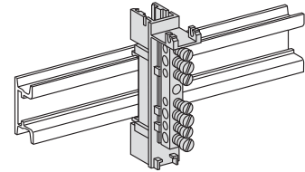
Монтаж клеммника на DIN-рейки
