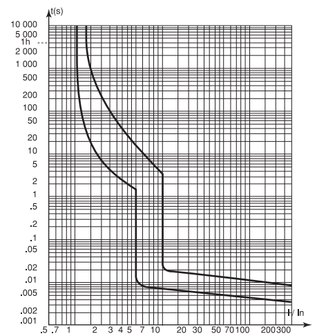
DPN, кривая С
