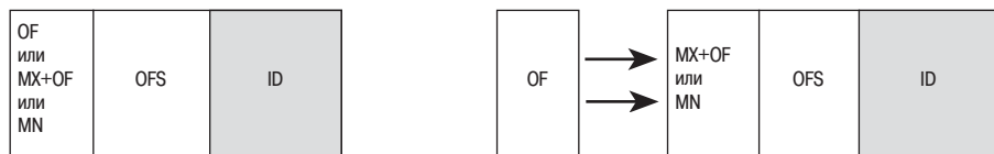
OF Блок-контакт состояния MX Независимый расцепитель MN Расцепитель минимального напряжения OFS (OFSP) Блок-контакт (обязателен) ID Дифференциальный выключатель нагрузки
