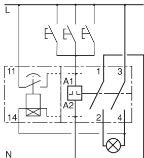
Таймер ATLt + импульсное реле TL
