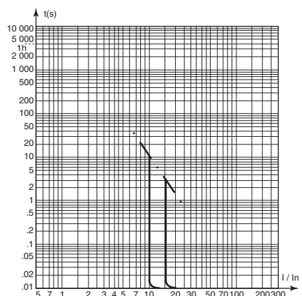
С60, кривая MA
