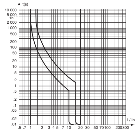
С60, кривая D
