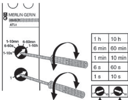
Настройка таймера ATLt
