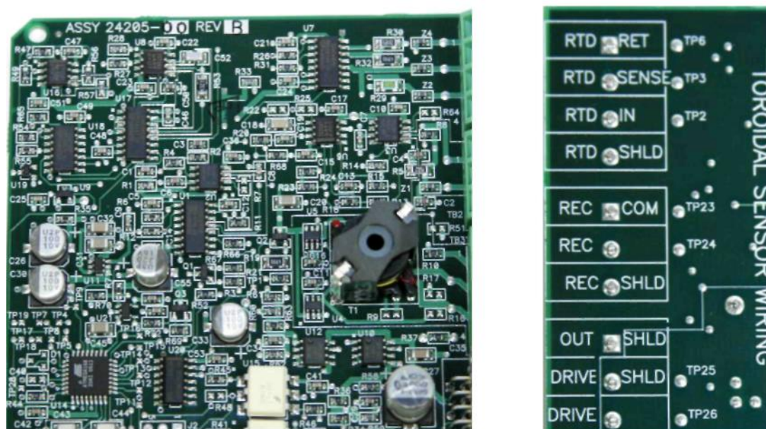
Рис. 3-7. Плата ввода сигналов от торoidalного датчика электропроводности и выводы кабеля датчика
