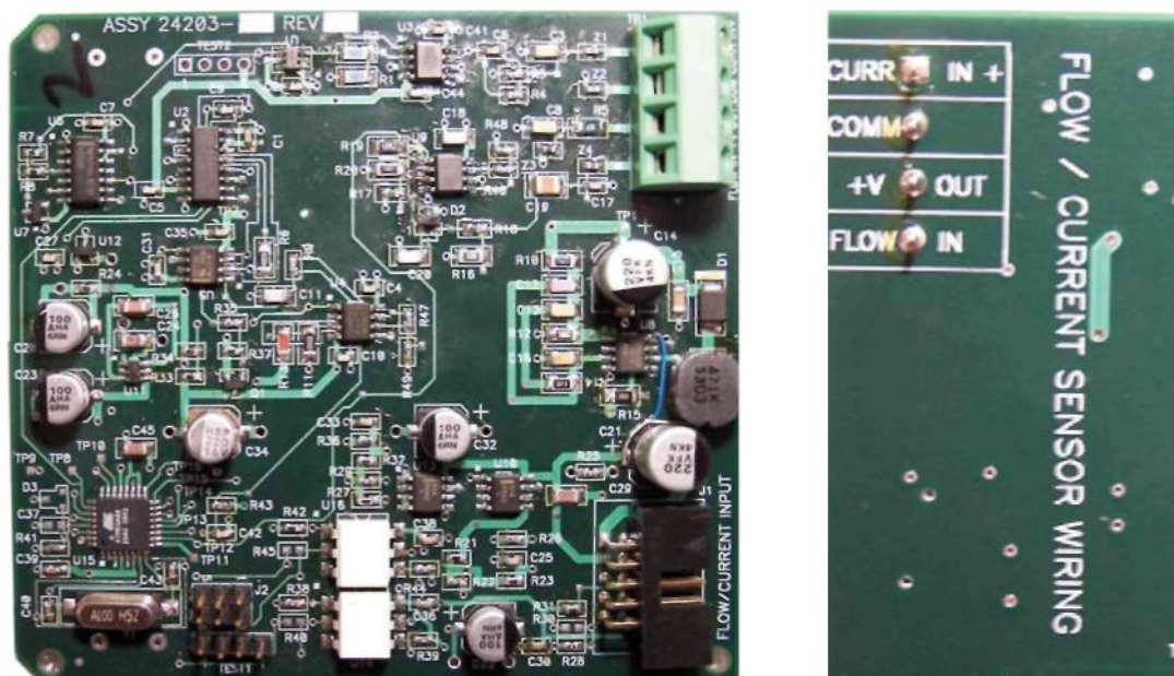
Рис. 3-11. Плата ввода сигналов расхода / токовых входных сигналов и выходы кабеля датчика
