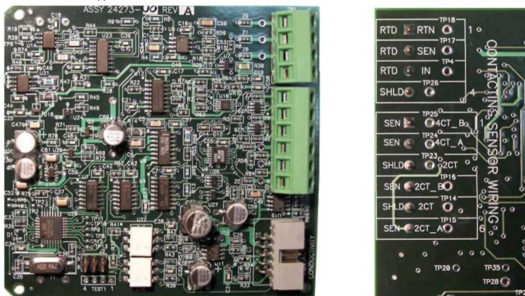
Рис. 3-6. Плата ввода сигналов от контактных датчиков электропроводности и выводы кабеля датчика
