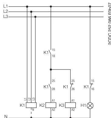
Схема цепи управления (K1 = CM-MPS.x3 или CM-MPN.x2)
