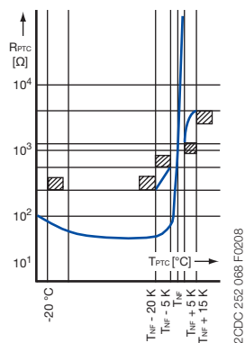
Кривая термометрических датчиков
