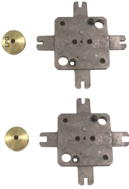
1- Content KITGPL 3122302 (KITGN 3142814) : n° 1 nozzle, n° 1 aluminium front part.
