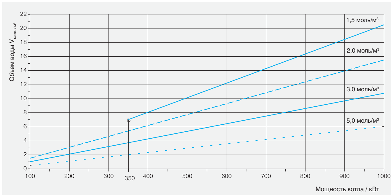
Расчетный объем воды V_{\text{макс}} для котлов \dot{Q} > 100 кВт до \dot{Q} = 1000 кВт и различных концентраций \text{Ca}(\text{HCO}_3)_2 , моль/м³
