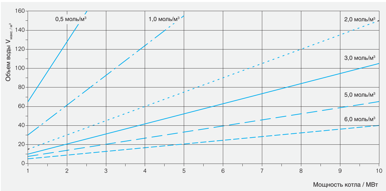
Расчетный объем воды V_{\text{макс}} для котлов \dot{Q} > 1 МВт до \dot{Q} = 10 МВт и различных концентраций \text{Ca}(\text{HCO}_3)_2 , моль/м³
