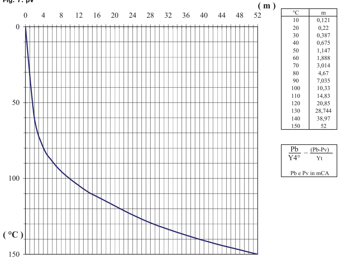
Fig. 7: pV
