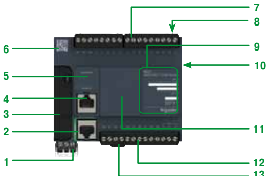
M221: 24 входа/выхода
