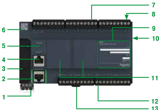
M221: 40 входов/выходов
