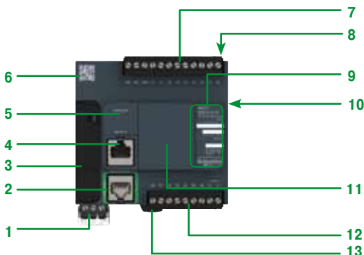
M221: 16 входов/выходов
