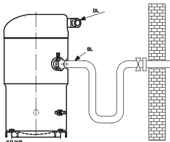
Рис 8: Конструкция всасывающего трубопровода
