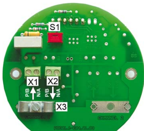
рис. 18: Плата подключения (стандартное исполнение)
