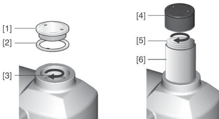
рис. 47: Пустотелый вал/шток
