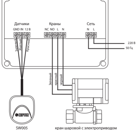
Рис.2 Схема подключения кранов шаровых с электроприводом серии НС 220 В к модулю управления Neptun Base
