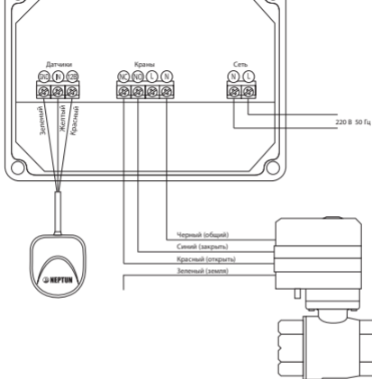
Рис. 4 Схема подключения кранов с электроприводом серии JW5000 220 VAC к модулю управления Neptun Base
