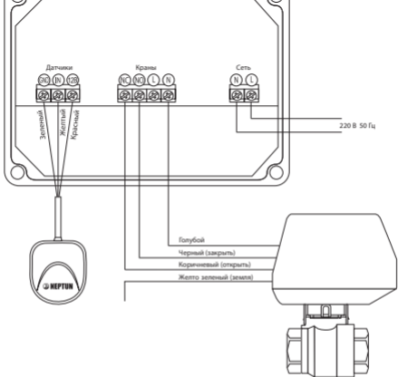
Рис. 3 Схема подключения кранов шаровых с электроприводом DePaLa 220 В к модулю управления Neptun Base
