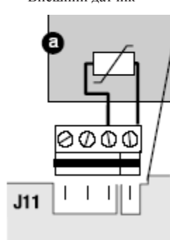
Внешний датчик
