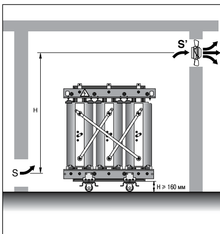
Принудительная вентиляция
