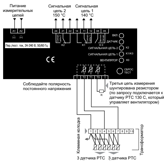
Схема соединений Z-преобразователя
