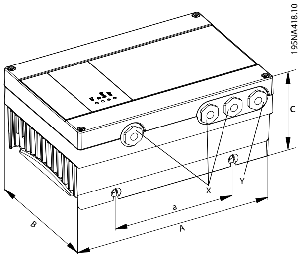
Рисунок 7.2 Размеры FCP 106
