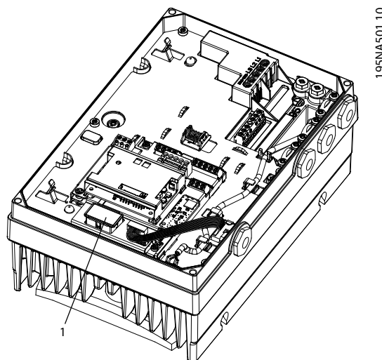
1 Модуль памяти VLT® Memory Module MCM 101
