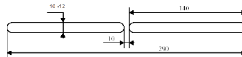
Размеры паза в раме створке/ раме окна
