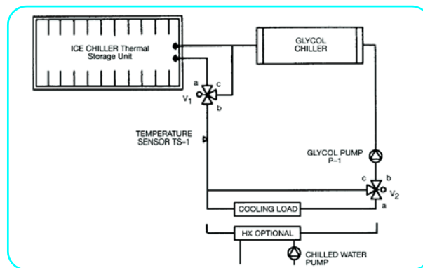
Одна насосная петля - охладитель перед накопителем
