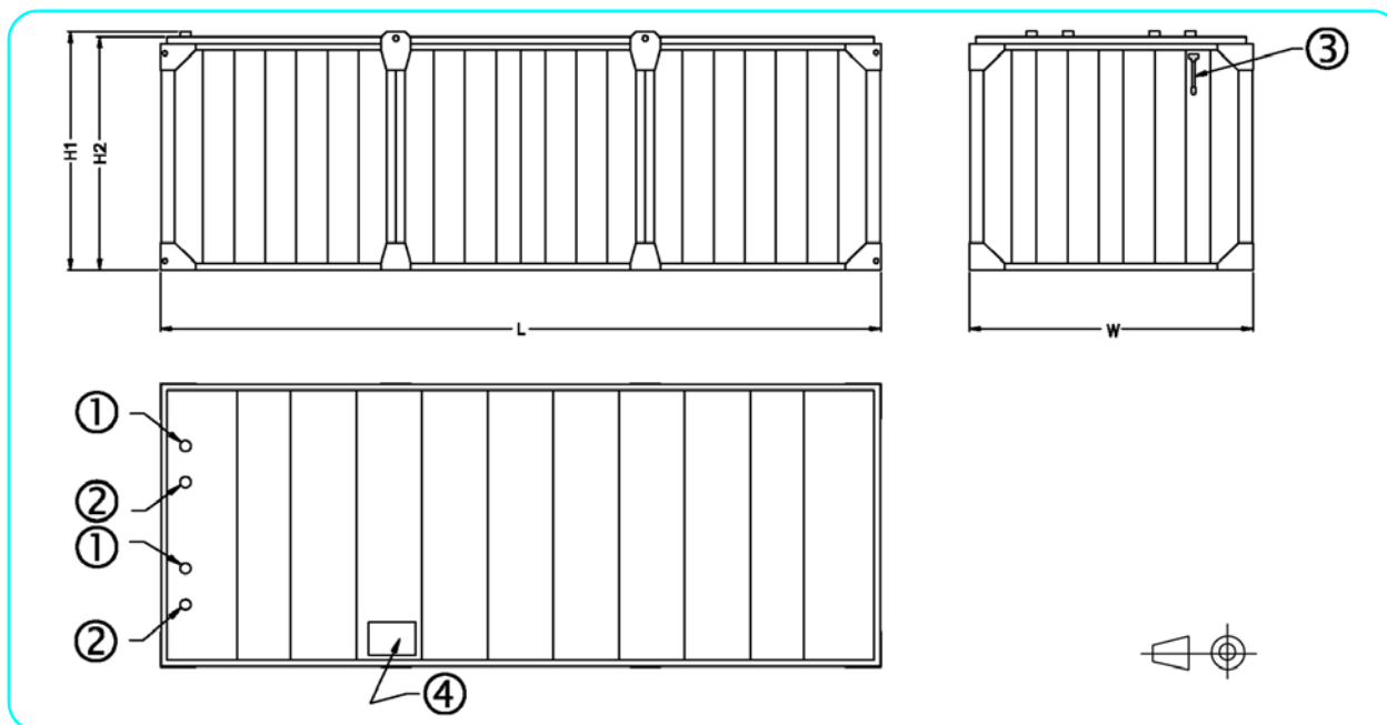
1. Выпуск; 2. Впуск; 3. Смотровая трубка; 4. Люк доступа.
