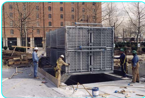
Монтаж модуля змеевика
