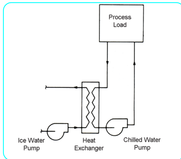
Схема с промежуточным теплообменником
