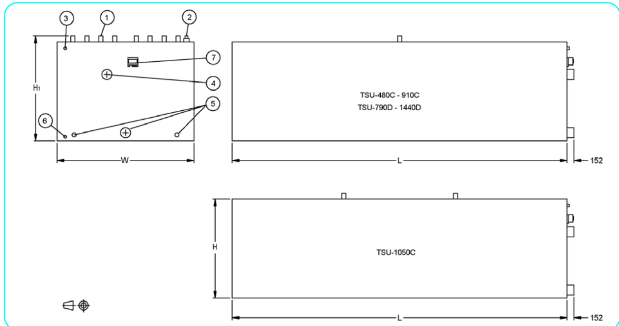
1. Соединители теплообменника; 2. Подпитка НД 50; 3. Перелив НД 50; 4. Выпуск воды; 5. Подача воды; 6. Слив НД 50; 7. ICE LOGIC®.
