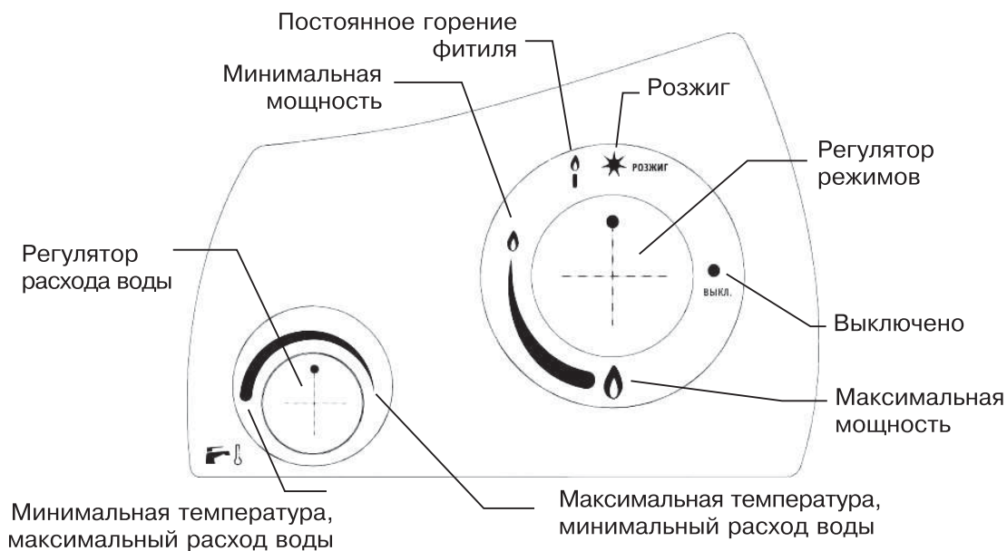
Рисунок 1. Панель управления водонагревателей серий S
