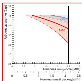
График насосов M10/D10
