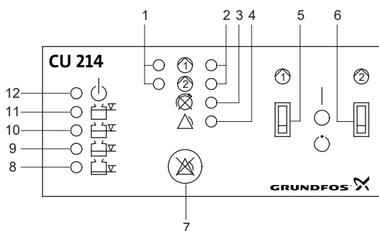
Рис. 23 Пульт управления модуля CU 214
