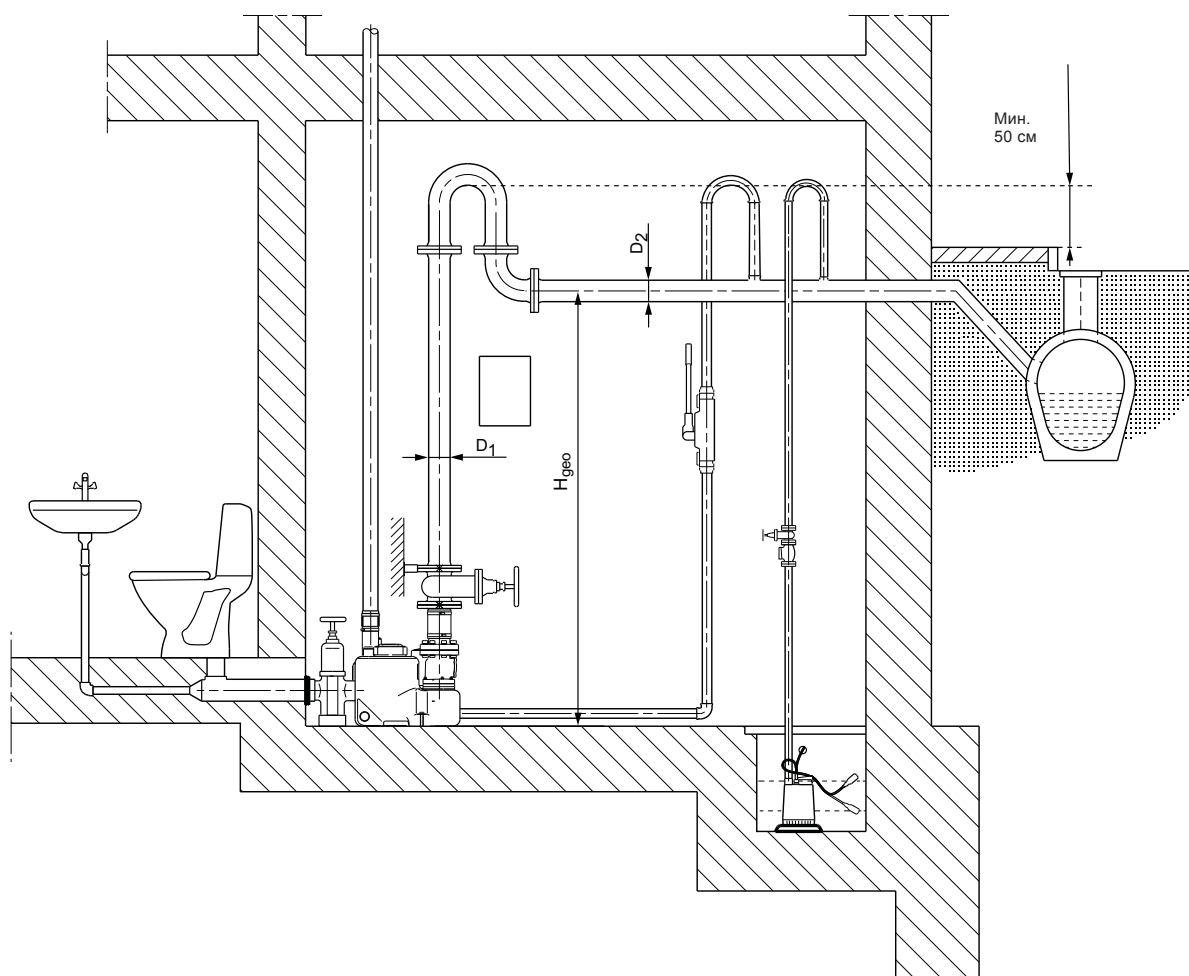
Рис. 5 Схема монтажа
