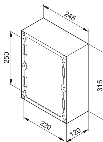
Рис. 11 Электрошкаф системы управления, предназначенный для настенного монтажа.
