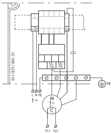
Рис. 18 Схемы электрических соединений
