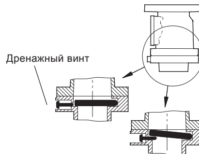
Рис. 19 Дренажный винт
