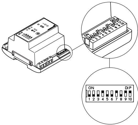
Рис. 21 Модуль CU 211 с микропереключателем
