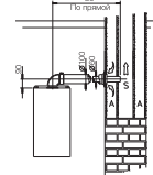
Горизонтальный коаксиальный дымоход
