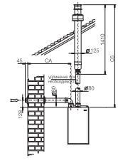
Раздельная система воздухозабора и вертикальным дымоотводом.
