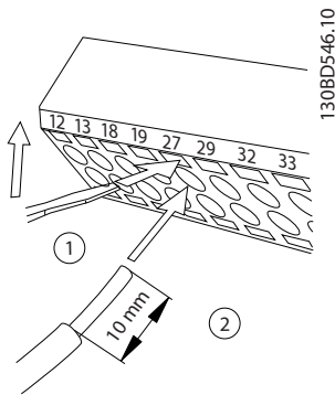
Рисунок 4.12 Подключение проводов цепи управления
