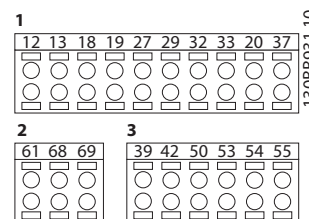
Рисунок 4.11 Номера клемм
