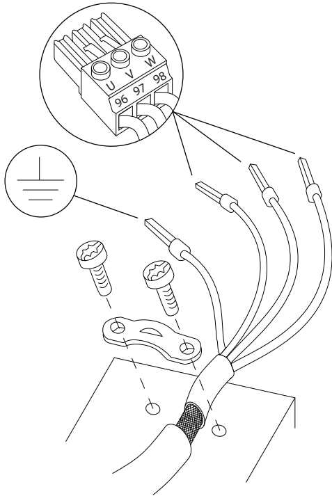
Рисунок 4.5 Подключение двигателя
