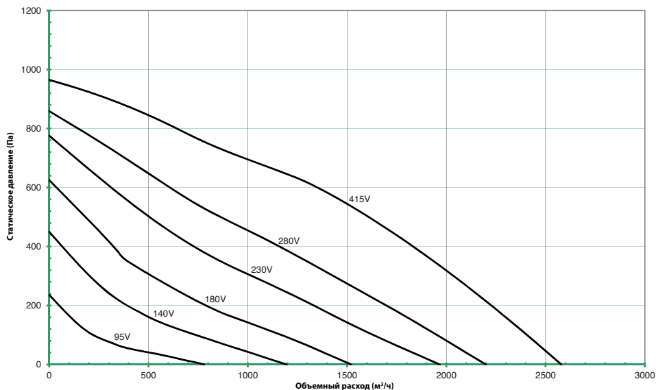
КАТANA 315-4-1(A)
