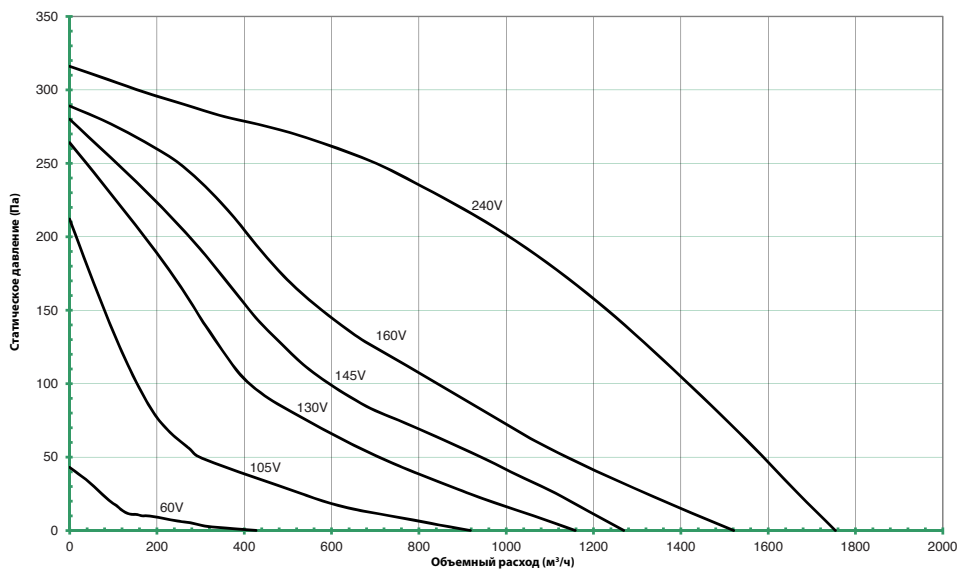
КАТANA 315-4-3 (A)
