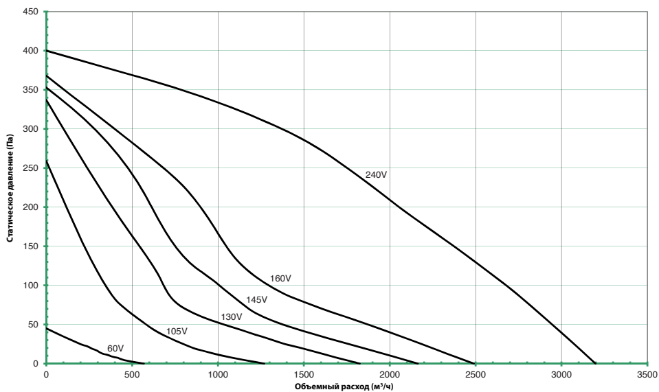
КАТANA 355-4-3 (A)
