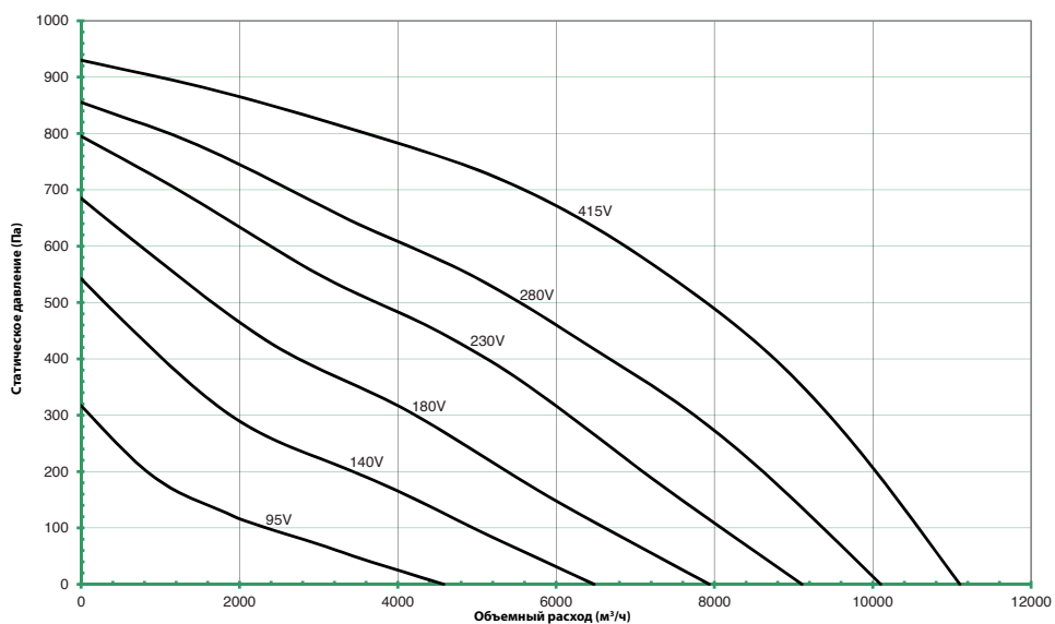
КАТANA 560-4-3 (A)
