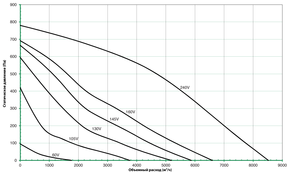
КАТANA 500-4-3 (A)
