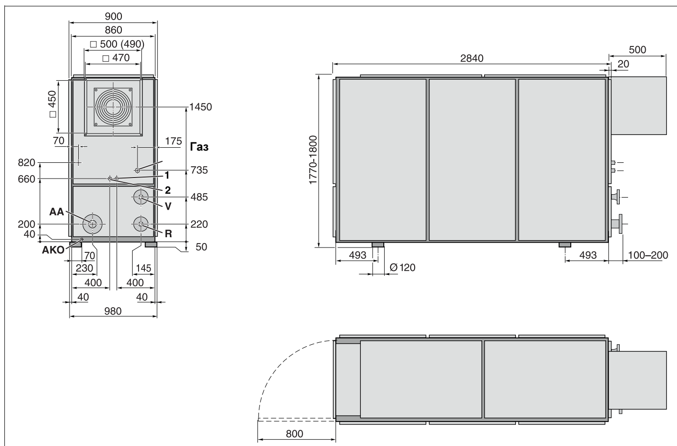
Рис. 4 Размеры (мм)
