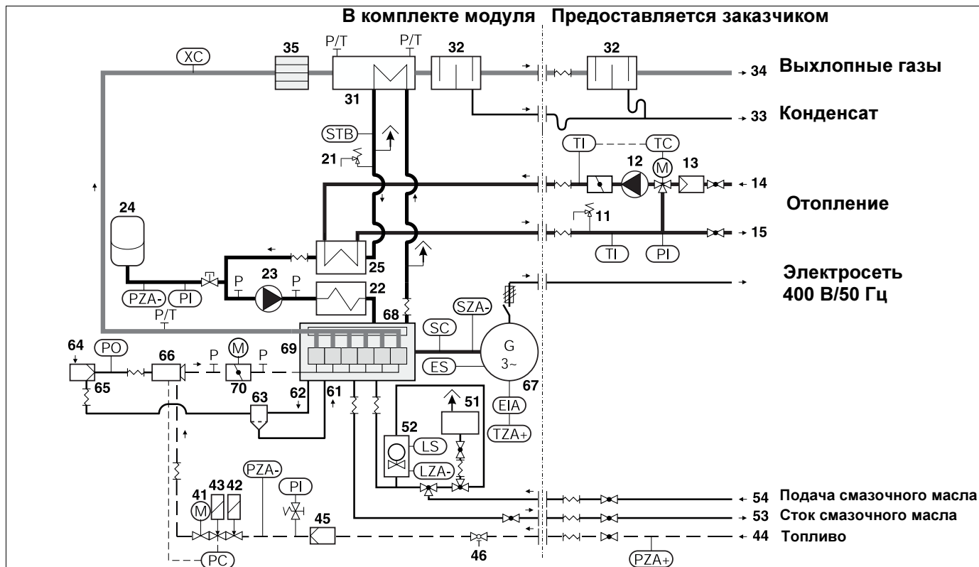
Рис. 2 Устройства контроля
