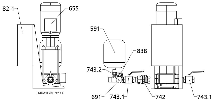
Рисунок 3: Общий вид Hya-Solo с Movitec 2, 4, 6, 10
