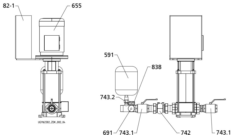
Рисунок 4: Общий вид Hya-Solo с Movitec 18
