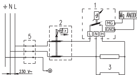
Электросхема
