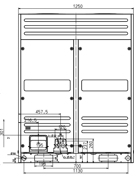
увеличенный вид для 18HP
