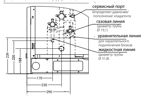
увеличенный вид для 18HP
