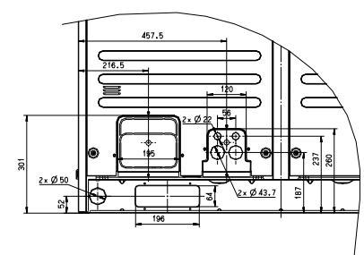
увеличенный вид для 12HP/14HP/16HP
