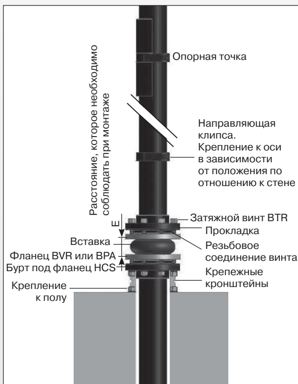
ВЕРТИКАЛЬНЫЙ МОНТАЖ
