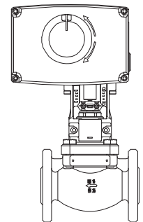
AME 25/AME 35 + VFS2 Д у 15–50
