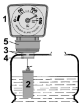
Рисунок 3: Сборка
